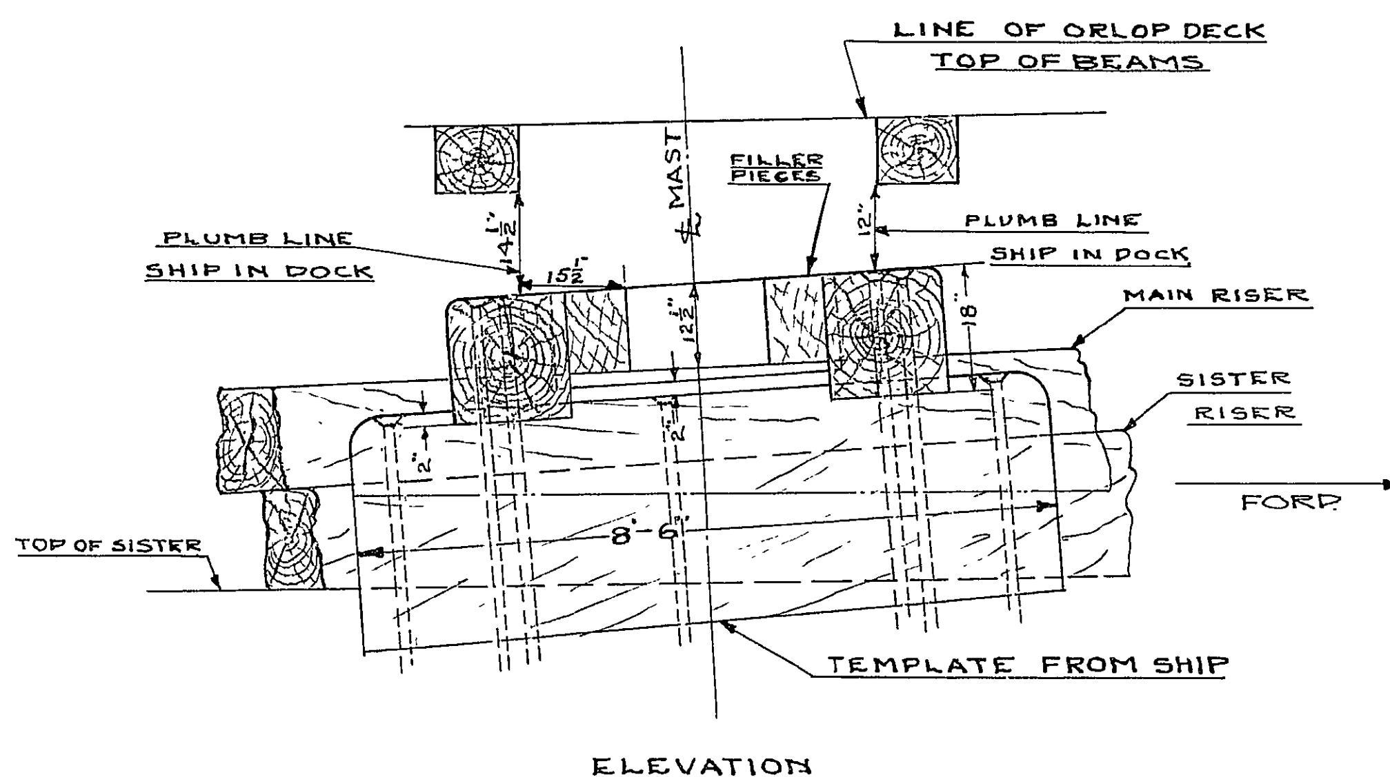
ELEVATION
